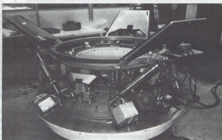
Dockningssektionen till den ryska sidan av dockningsmodulen.
