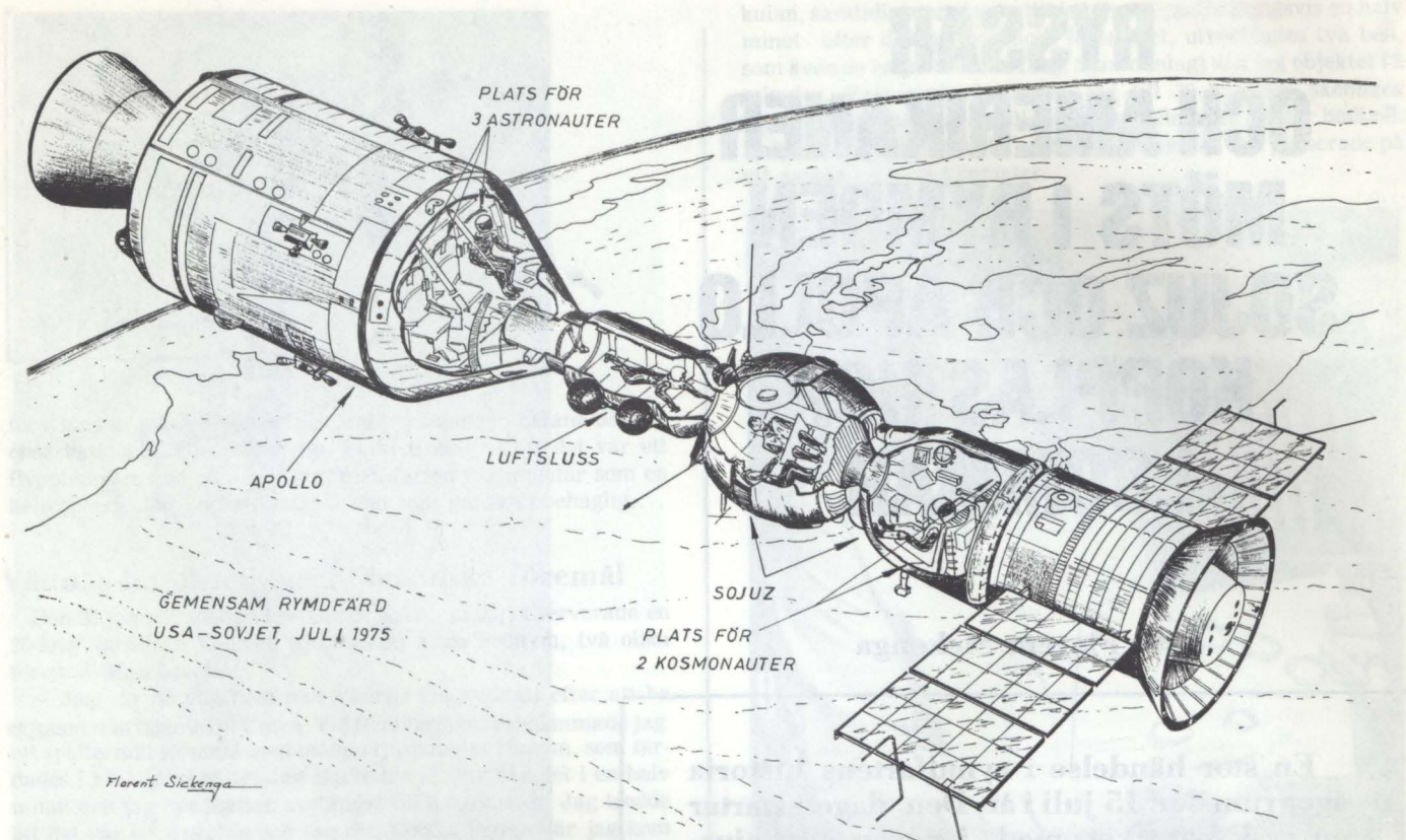
Apollo och Sojuz sammankopplas i rymden. I mitten ses luftslossen, även kallad dockningssektion. Apollokapseln bjuder plats åt tre, Sojuz åt två rymdmän.
